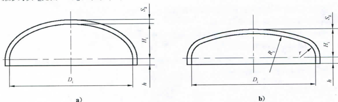
图 1 封头形状示意图
