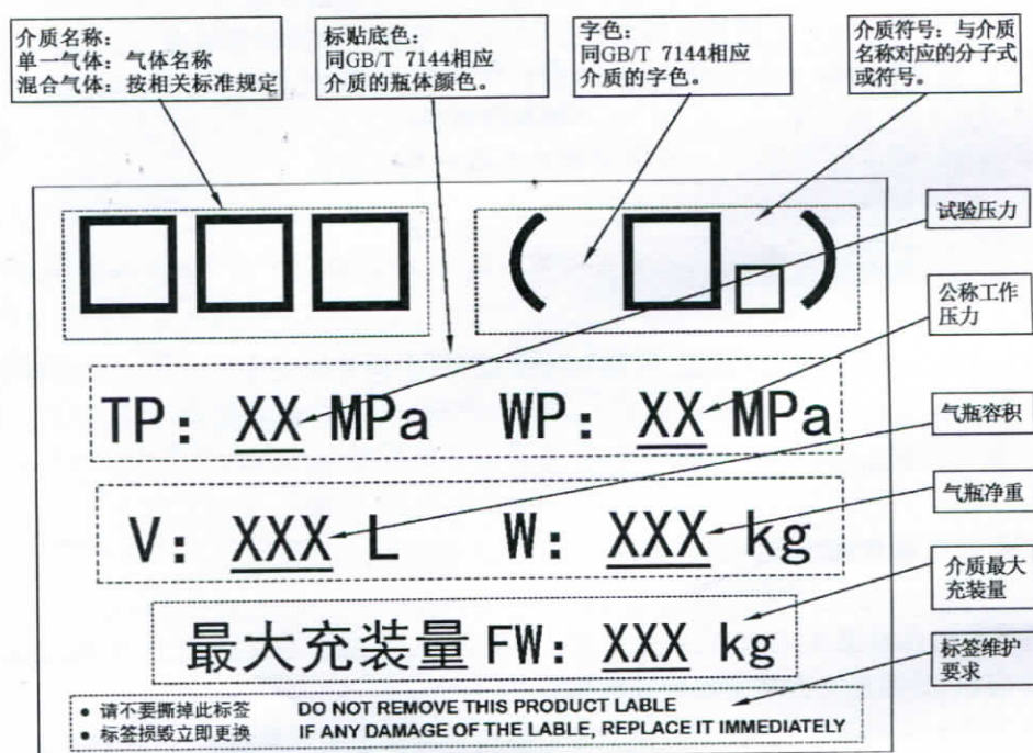
图 A.1 介质标贴示意图
