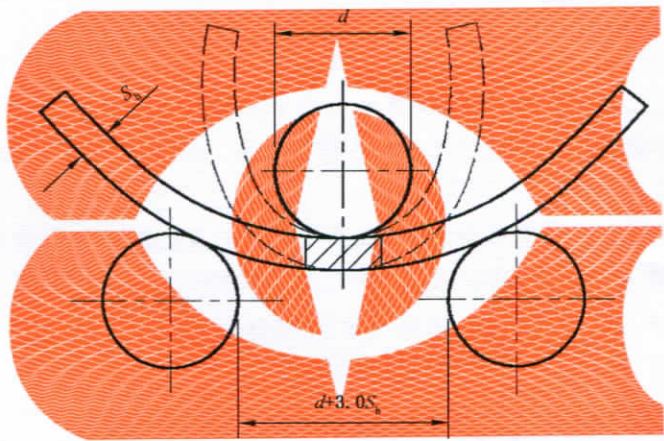
图 11 弯曲试验示意图
