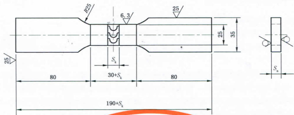
图 10 拉伸试样图
