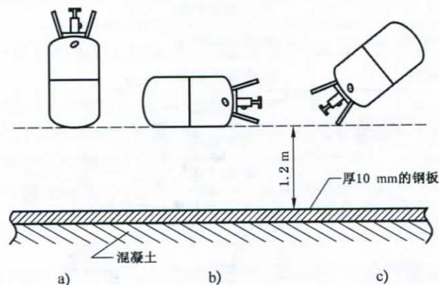
图 A.2 跌落试验
